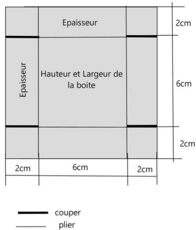
Gabarit interieur de la boîte
